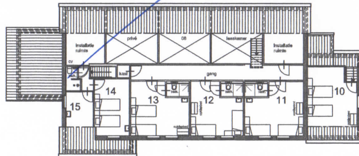
plattegrond verdieping
