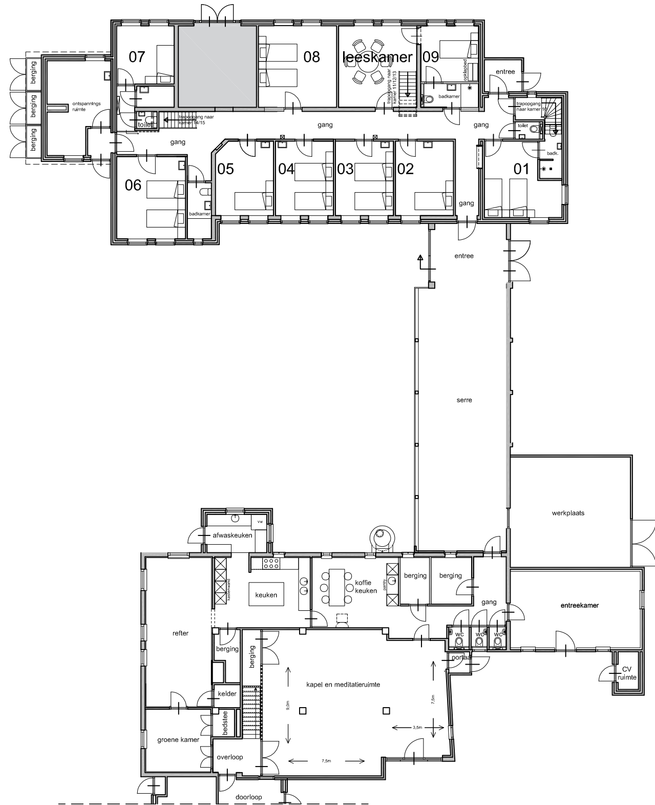
plattegrond begane grond
