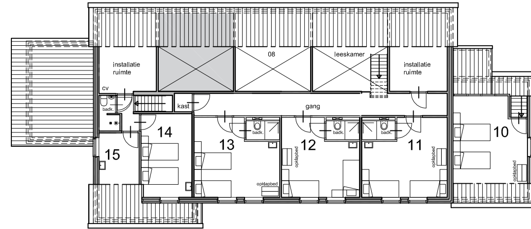
plattegrond verdieping
