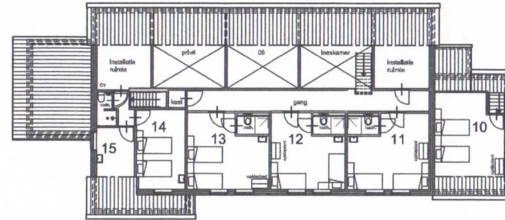
plattegrond verdieping
